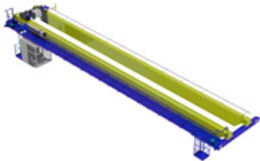
Кран мостовой электрический двухбалочный
